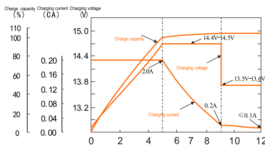
Charge characteristics 77°F (25°C) / Caractéristiques de charge 77°F (25°C)
